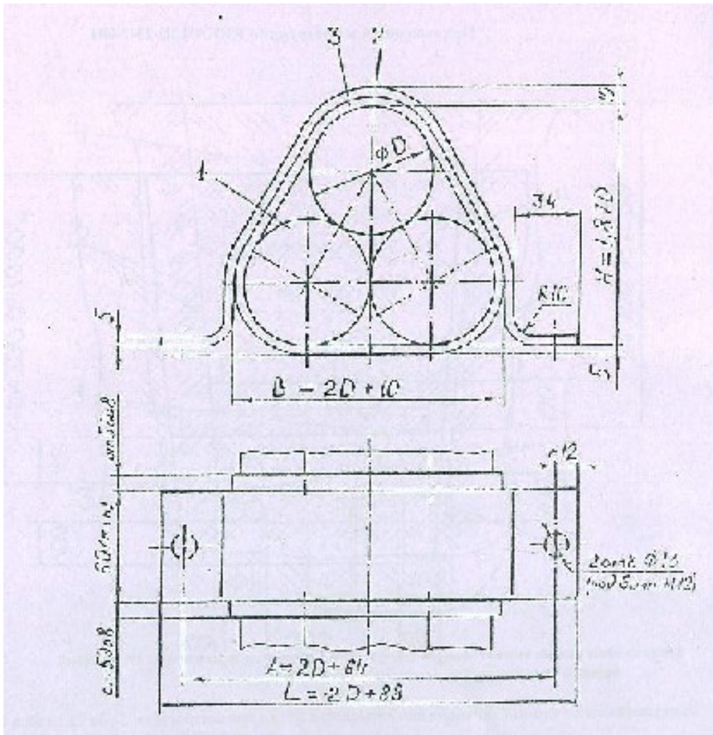
Рисунок 3. Крепление трёх кабелей в связке на металлоконструкции (вариант исполнения)
